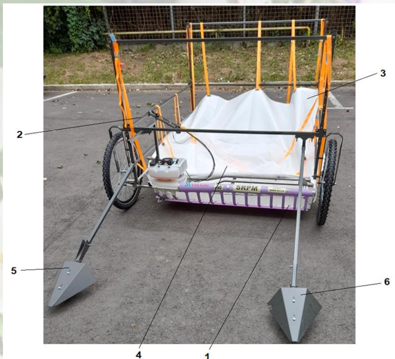
Fig. 1. Sistemul tehnic de recoltat plante medicinale SRPM
